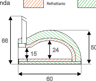
Sezione trasversale
